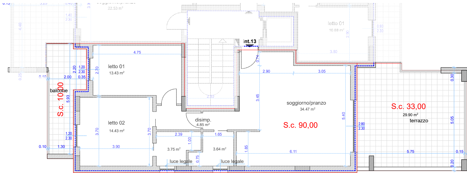
PLANIMETRIA QUOTATA
