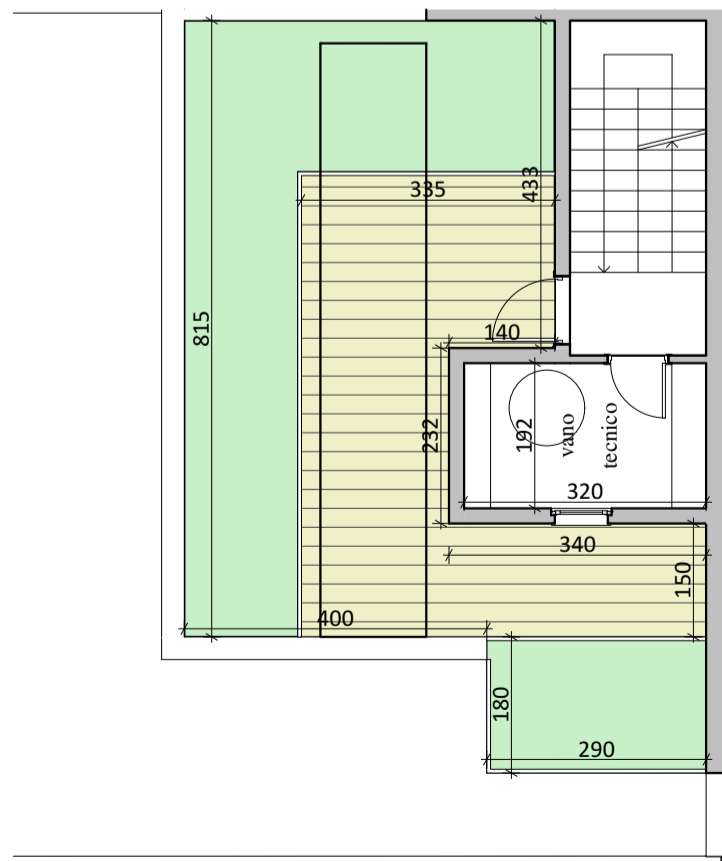
Pianta piano copertura
